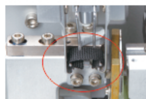
自动折边装置 Automatic folding device
